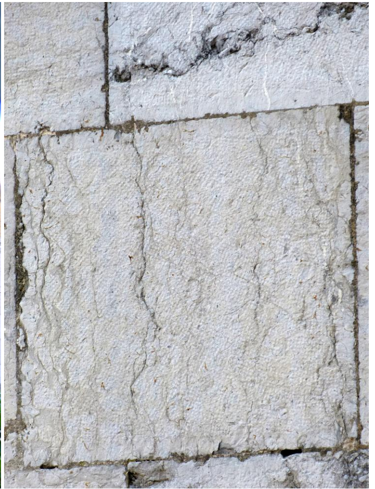
stylolythes sur l'église St Laurent
