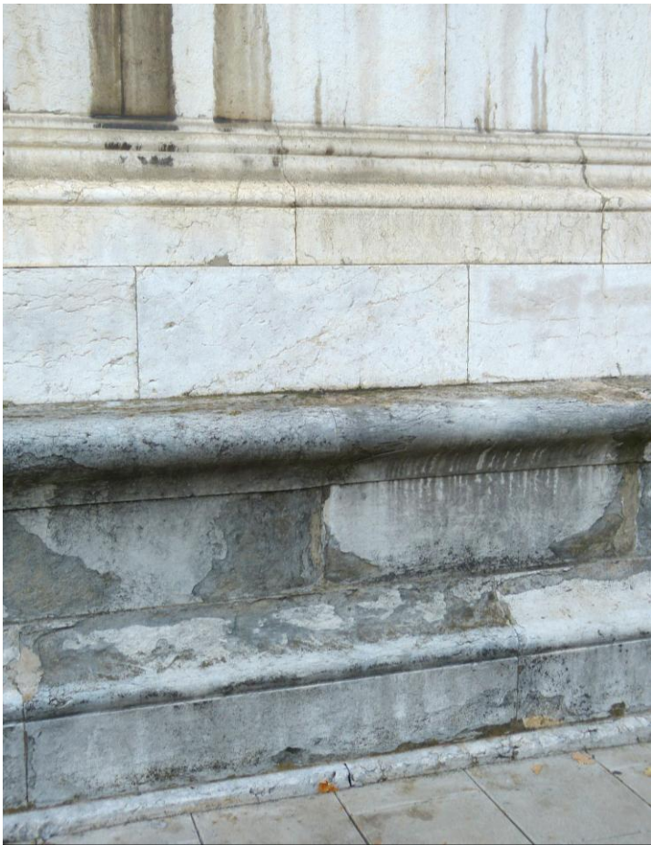
Ancien musée de peinture : tithonien et urgonien
